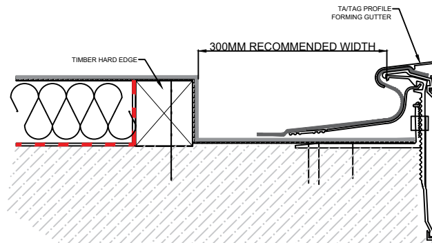
TA/TAG GUTTER
